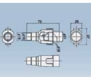
DHB-1416 Vannlås for kondensvannrør
