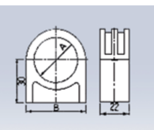
NDH-14S, kobling mellom slange DH-14 og rør ND-20
