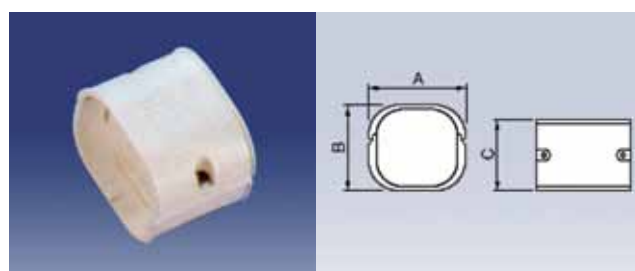
SJ, mufte
