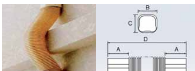
SF, flexibel kanal
