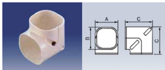
SCM, kort albue 90 grader
