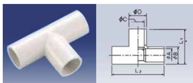
NDT-20, T-rør
