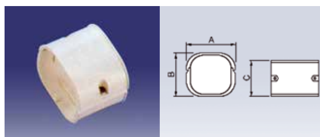
SJ, muffe
