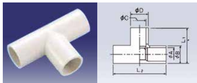
NDT-20, T-rør
